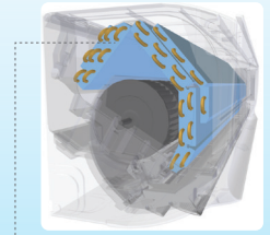
Heat Exchanger Current Inverter Permukaannya memiliki suhu yang sama
