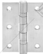
ESS EL 3X2,5X2MM 2BB SSS Capacity (max) : 30 KG / pair
