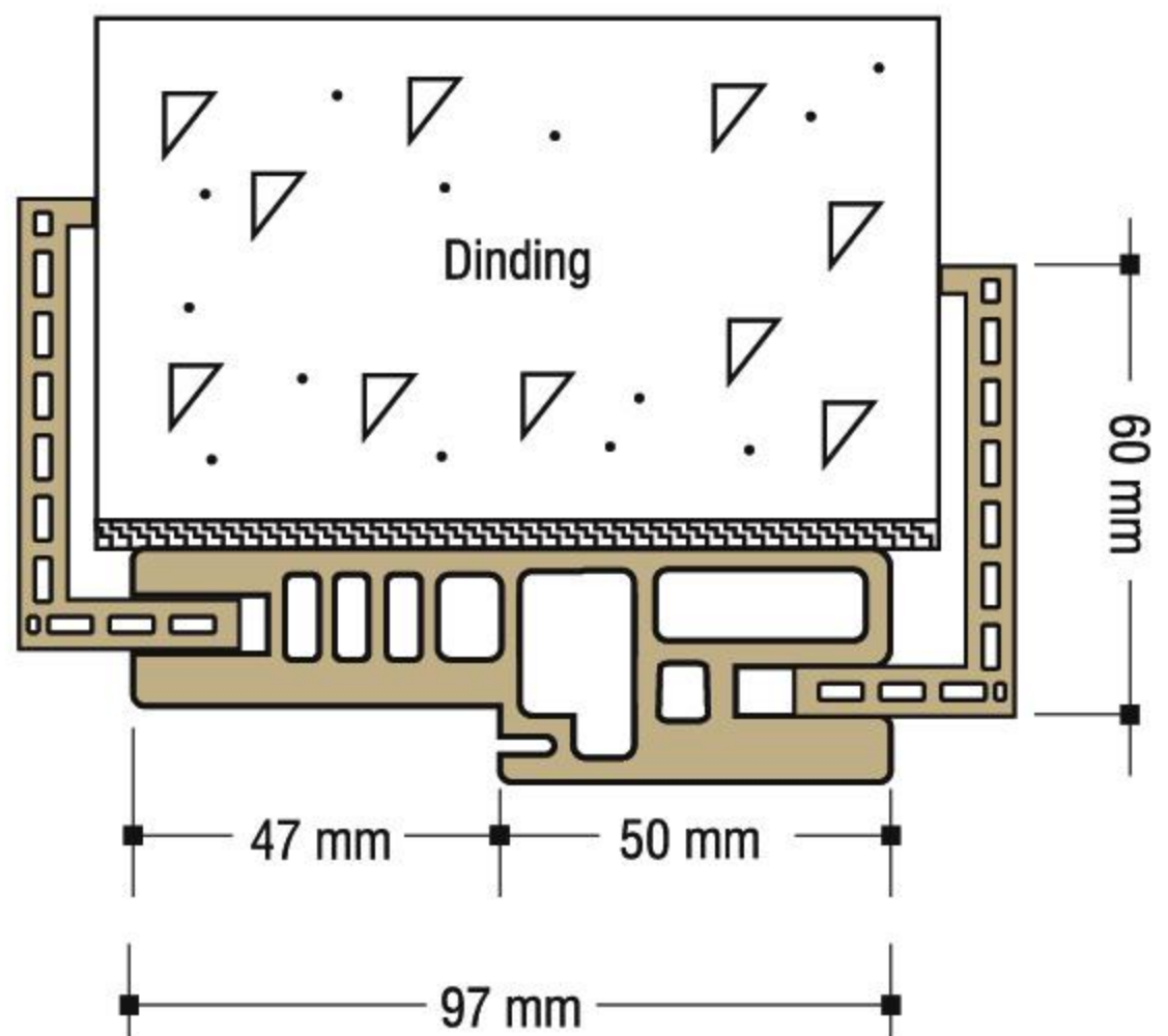
Ilustrasi Pemasangan Kusen + Architrave
