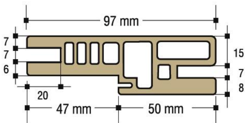
Gambar Profil Kusen
