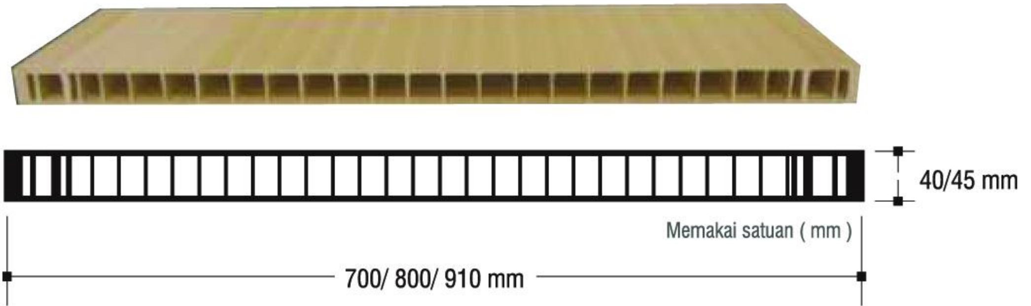
Gambar Profil Pintu
