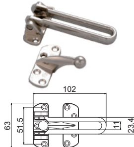
Door Stopper B 29
