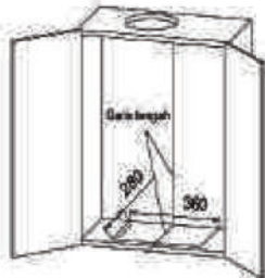
Ukuran Lubang Bukaan Langit Langit atau Atas Kabinet. Ukuran Lubang Bukaan Lantai Kabinet
