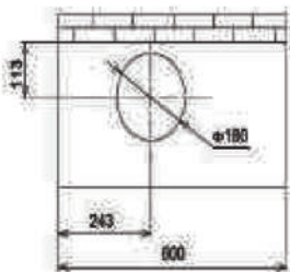
Ukuran Lubang Bukaan Langit Langit atau Atas Kabinet. Ukuran Lubang Bukaan Lantai Kabinet
