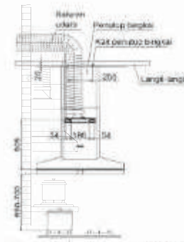
Gambar 2. Skema pemasangan
