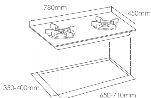
Hob GHG78211
