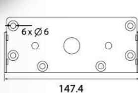
Roda Atas Bagian Dalam 1 Set Kiri dan Kanan
