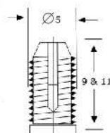
Fisher FIS-59 5 x 9 mm (Merah) FIS-512 5 x 12 mm (Putih)
