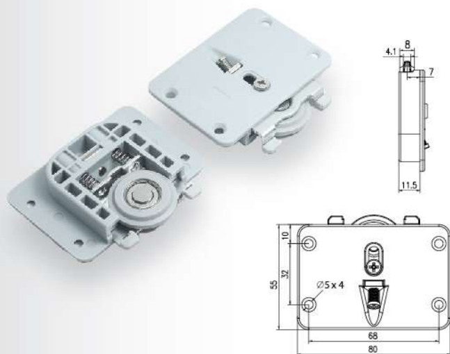
SD-451 (1 Pintu) Roda Atas (Plastik) : 2 Pcs SD-452 (2 Pintu) Roda Atas (Plastik) : 4 Pcs
