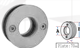
Material : Stainless Steel Sus 304 Type : HT 2450 Size A : 36 mm, Size B : 75 mm
