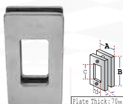
Material : Stainless Steel Sus 304 Type : HT 2462 Size A : 69 mm, Size B : 121 mm
