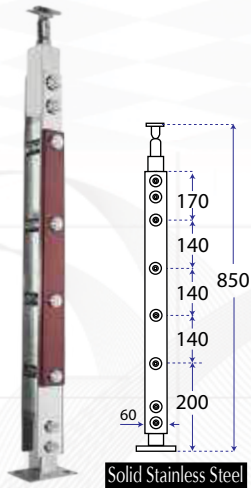
Type : RT 0119 Finish : Ch (Chrome) Material : SS SUS 304 + Wood Description : Hand-Rail for Pipe
