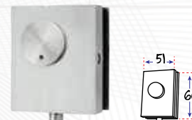
Glass Door Bolt ~sn Type : APL 0001 Material : Stainless Steel Sus 304
