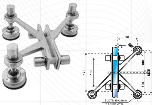
Type : BX 8318 Side : R (Right) 45° Material : Stainless Steel Sus 304
