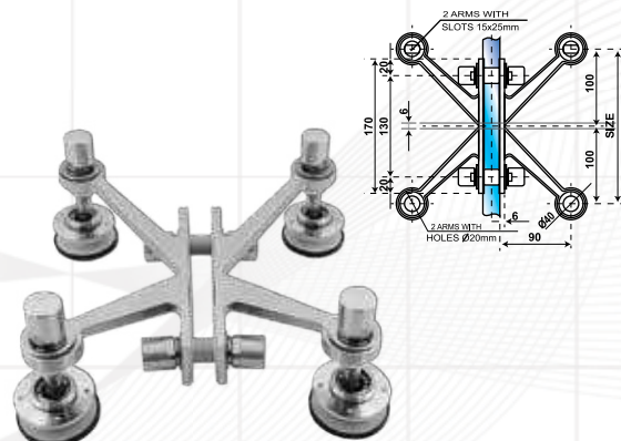
Type : BX 8319 Size : 200 mm Material : Stainless Steel Sus 304
