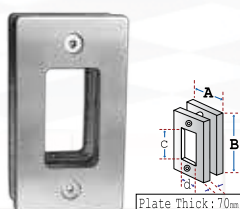
Material : Stainless Steel Sus 304 Type : HT 2463 Size A : 69 mm, Size B : 121 mm
