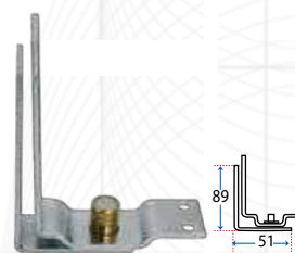
Bottom Pivot Folding Door
