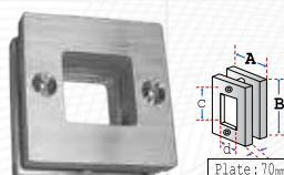
Material : Stainless Steel Sus 304 Type : HT 2452 Size A : 75 mm, Size B : 75 mm
