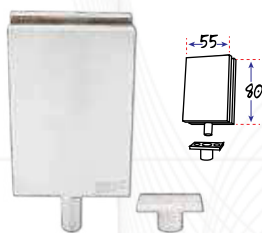
Bottom Pivot RDG BP 5700 ~sn Type : SP 8206 Material : Stainless Steel Sus 304 Max Weight : 80 kg/door leaf
