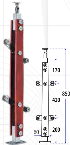
Type : RT 0101 Material : SS SUS 304 + Wood Description : Hand-Rail for Glass
