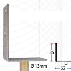
Folding Door Guide (L)
