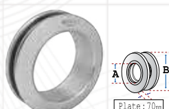
Material : Stainless Steel Sus 304 Type : HT 2451 Size A : 38 mm, Size B : 63 mm
