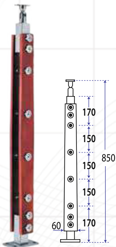
Type : RT 0100 Material : SS SUS 304 + Wood Description : Hand-Rail for Pipe
