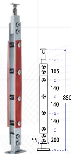
Type : RT 0113 Material : SS SUS 304 + Wood Description : Hand-Rail for pipe
