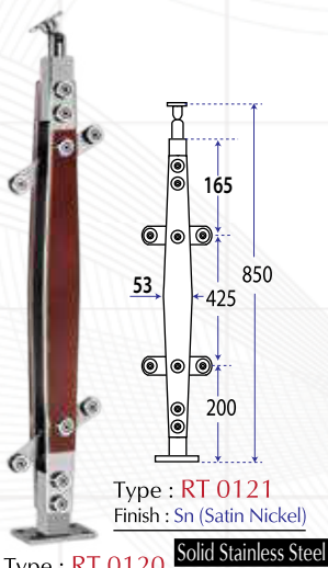
Type : RT 0120 Finish : Sn (Satin Nickel) Material : SS SUS 304 + Wood Description : Hand-Rail for Glass
