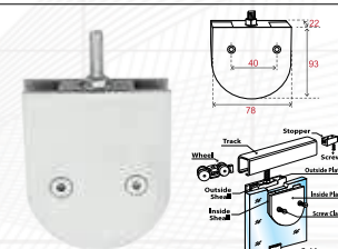
Sliding Glass Door Clamp
