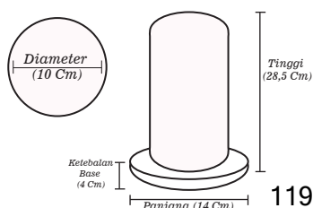
Original Lampu Pilar/Taman 1726-280-BH E27 X 1 Aluminium & Kaca
