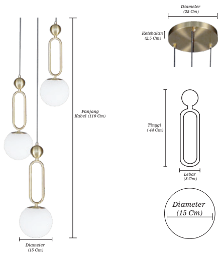
Original Lampu Gantung 9114-3 GD E.27X3 Berat Lampu 4 Kg Besi & Kaca
