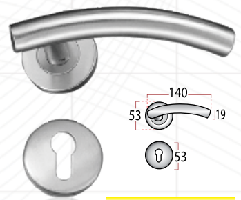
Type : HX 2156
