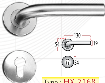
Type : HX 2168
