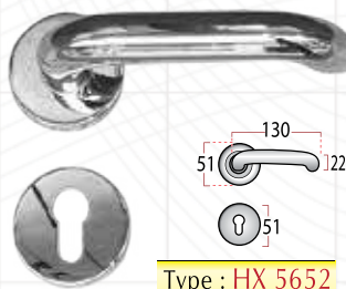
Type : HX 5652
