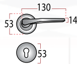
Type : HX 8622
