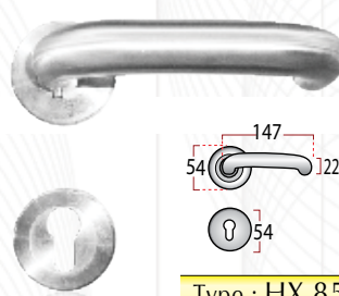
Type : HX 8519
