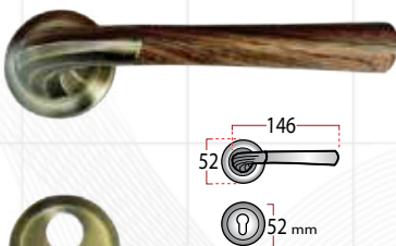
Type : HX 8501
