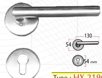
Type : HX 2190
