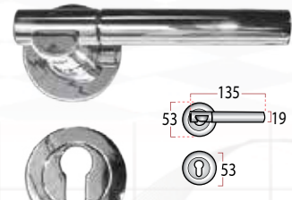
Type : HX 5676
