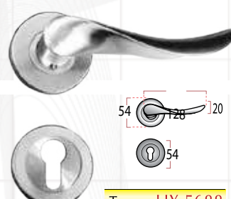
Type : HX 5688
