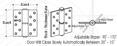
Door Closer Hinge
