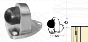
Type : DS 6424 Material : Zinc Alloy Description : Rubber Endure System
