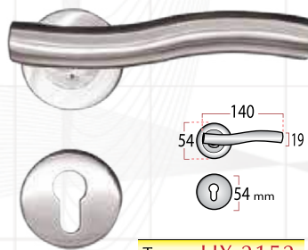
Type : HX 2152
