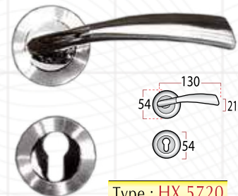
Type : HX 5720
