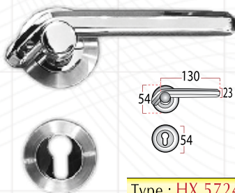
Type : HX 5724
