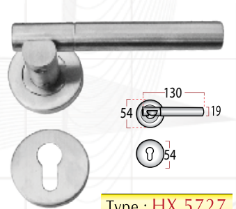
Type : HX 5727
