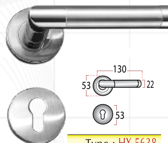
Type : HX 5638
