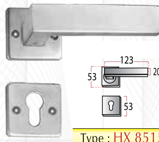
Type : HX 8515
