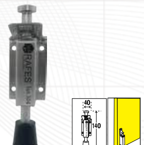
Type : New Arrival Material : Stainless Steel Sus 304 Description : Rubber Endure System
