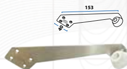
Type : DS 6454 Material : Stainless Steel (Sus 304)
