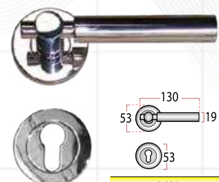
Type : HX 5697
