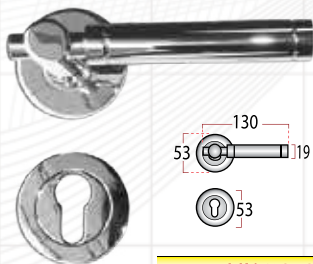
Type : HX 5673
