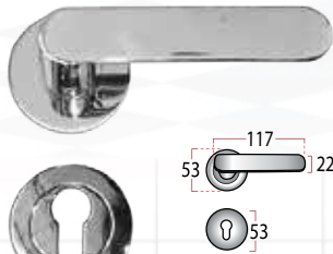
Type : HX 5674
