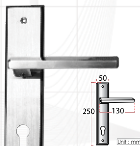
Type : HX 5660
