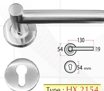
Type : HX 2154
