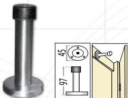
Type : DS 6422 Material : Stainless Steel Description : Rubber Endure System
