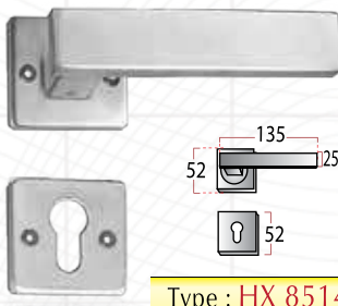
Type : HX 8514
