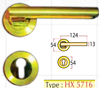
Type : HX 5716
