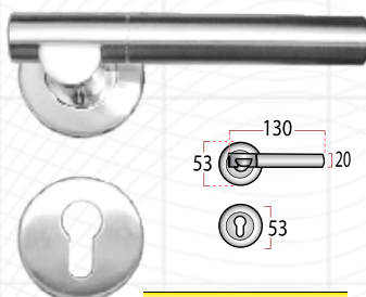
Type : HX 5737
