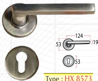
Type : HX 8573
