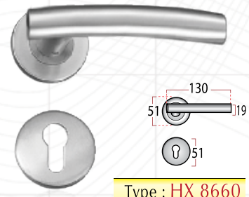
Type : HX 8660
