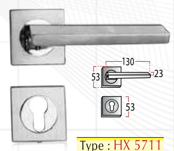
Type : HX 5711
