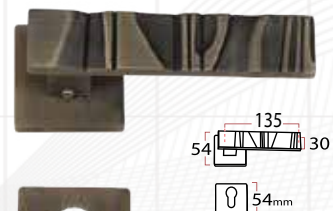
Type : HX 8538
