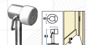
Type : DS 2637 Material : Stainless Steel Description : Rubber Endure System
