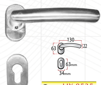
Type : HX 8535
