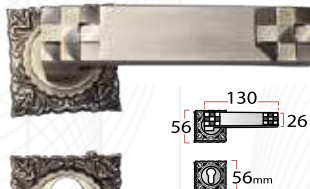
Type : HX 5796
