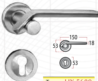
Type : HX 5689
