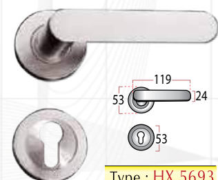
Type : HX 5693
