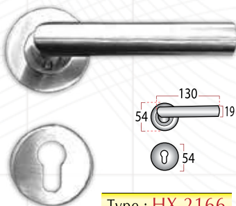
Type : HX 2166
