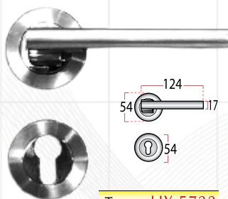
Type : HX 5722
