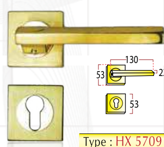
Type : HX 5709
