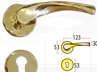
Type : HX 8678
