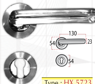
Type : HX 5723
