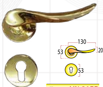
Type : HX 8677
