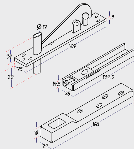
Type : PS 4000 Description : Floor hinge Rafes Bar
