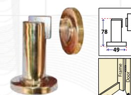
Type : DS 6428 Material : Stainless Steel (Sus 304) Description : Magnetic System
