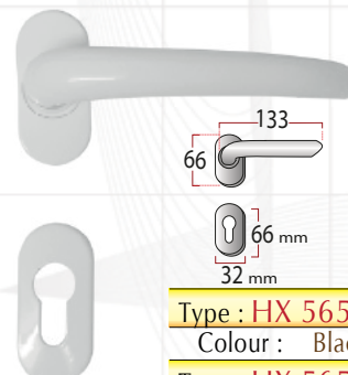
Type : HX 5654
