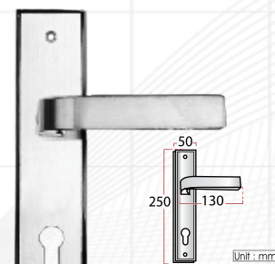
Type : HX 5665
