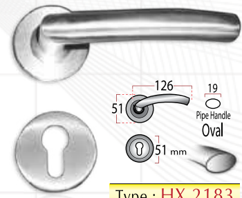
Type : HX 2183
