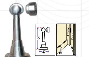
Description : Magnetic System Material : Stainless Steel Sus 304 Type : DS 6451 Type : DS 6453 Finish : Sn Finish : Ab
