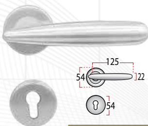
Type : HX 8551
