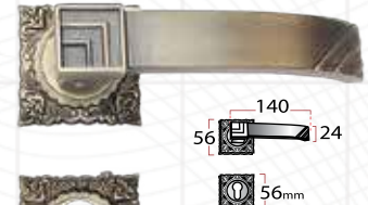
Type : HX 5797
