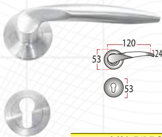
Type : HX 5758
