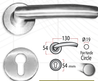
Type : HX 2158
