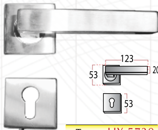
Type : HX 5730
