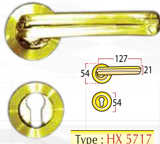
Type : HX 5717
