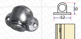
Type : DS 6342 Material : Stainless Steel Description : Magnetic System
