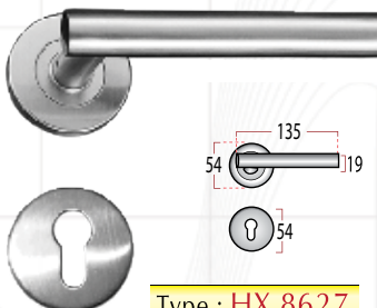
Type : HX 8627
