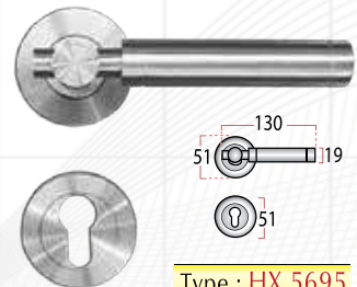
Type : HX 5695
