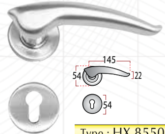
Type : HX 8550
