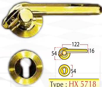
Type : HX 5718
