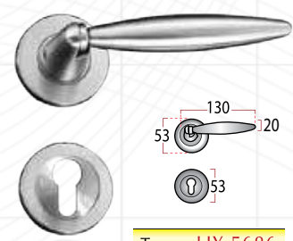
Type : HX 5686
