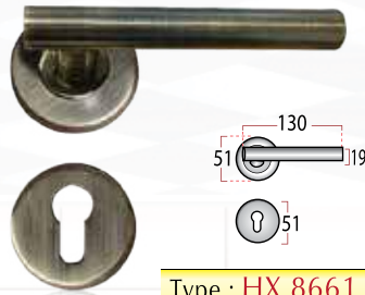
Type : HX 8661
