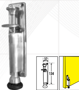
Type : DS 6415 Material : Stainless Steel Sus 304 Description : Rubber Endure System
