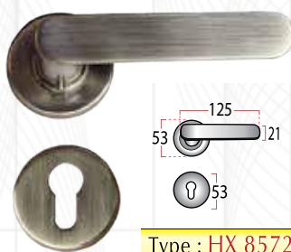
Type : HX 8572
