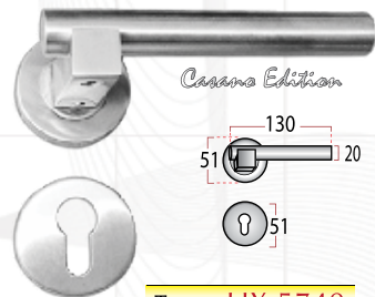
Type : HX 5740
