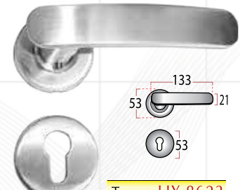
Type : HX 8623
