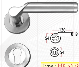
Type : HX 5678
