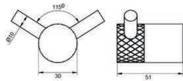
V-VT 5455 GY Double Hook • SUS 304 Body • Brass Engraved Head • Grey Colour
